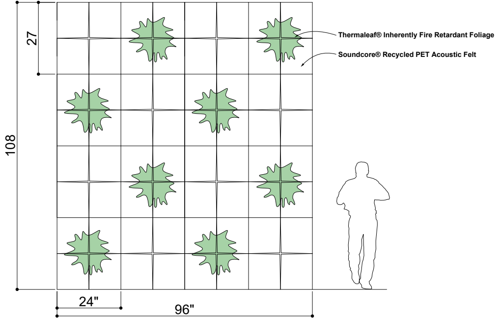
① ELEVATION 1
