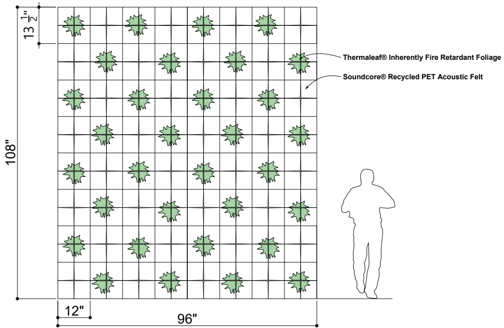
② ELEVATION 2
